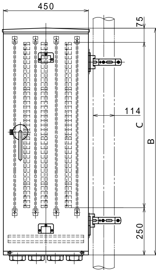
種別寸法表
