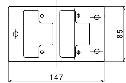
DCE 2個穴 (重量91g)
