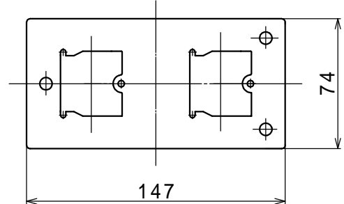
BM1004A 2個穴 (重量103g)
