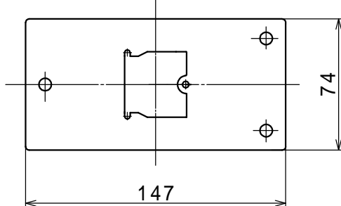
BM1004A 1個穴 (重量120g)
