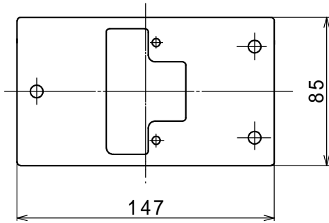
DCE 1個穴 (重量123g)
