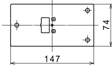
SM480 1個穴 SM1600 1個穴 (重量 130 g)
