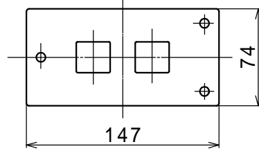
S600 2個穴 (重量 117 g)
