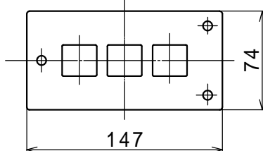
S600 3個穴 (重量 111 g)
