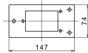
F形 1個穴 (重量 84 g)
