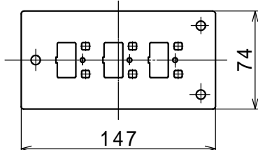
SM480 3個穴 SM1600 3個穴 (重量 115 g)
