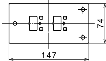
SM480 2個穴 SM1600 2個穴 (重量 120 g)
