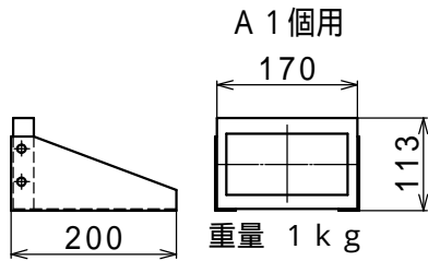
クッションゴム ゴムの高さ約10mm
