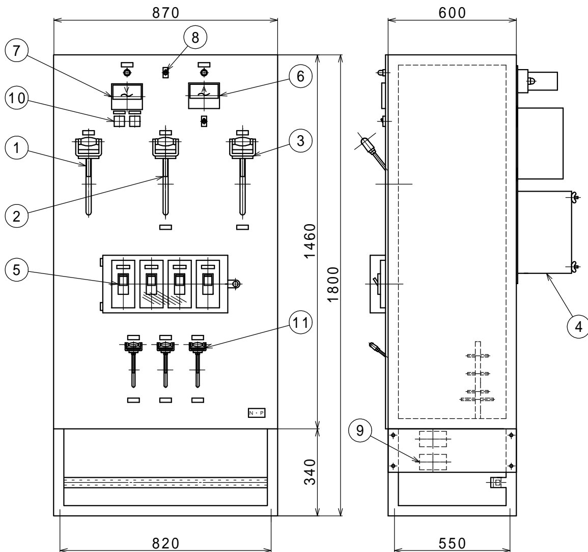
端子盤
