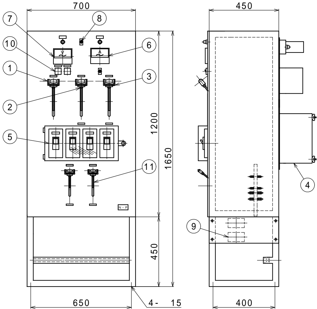
端子盤
