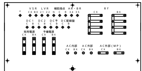
端子盤
