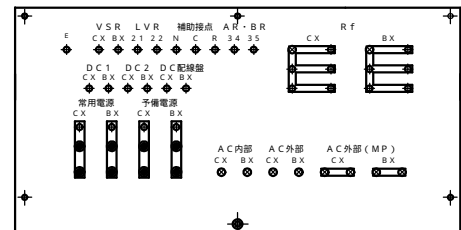
端子盤
